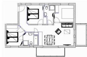
Grundriss
