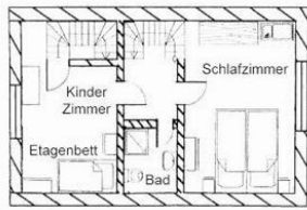
Grundriss 1. OG
